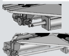
Verstellbares Spannsystem (Spannbereich 10" ÷ 27")
