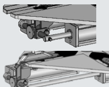
Système de verrouillage réglable (capacité 10" ÷ 27")
