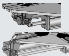
Sistema de cierre con mordazas ajustables (capacidad 10" ÷ 27")
