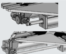
Verstellbares Spannsystem (Spannbereich 10" ÷ 27")
